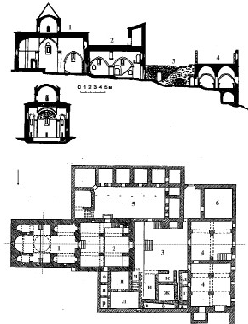
Рис. 3. Монастырь Сурб Хач. Общий план, продольный разрез храма, притвора, центрального двора, трапезной и поперечный храма (по В. А. Сидоренко): 1 – храм; 2 – притвор; 4 – трапезная; 5 – братский корпус с двориком; 6 – предвратный комплекс; 3 – центральный двор с строительными остатками, открытыми в 1973, 1976, 1979 г.
