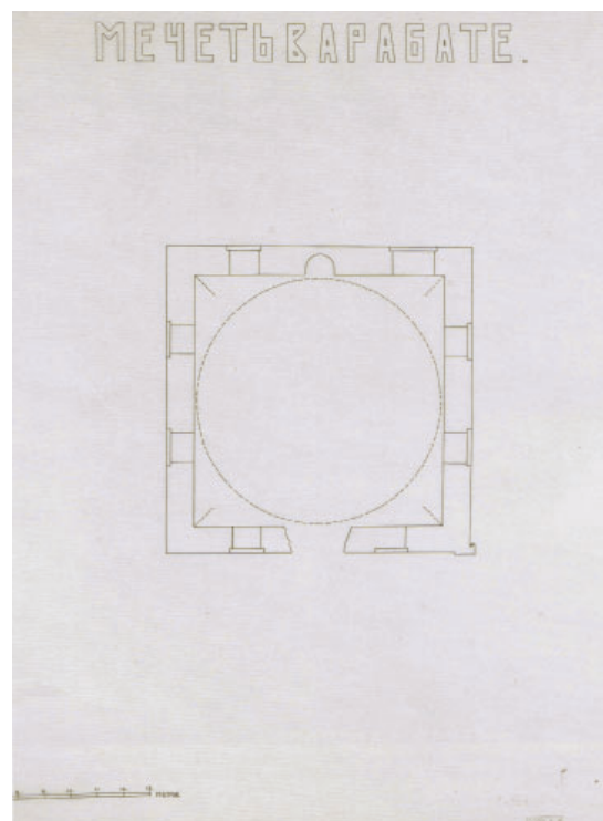
Рис. 4. План мечети крепости Арабат. Калька, тушь. 1928 г. Автор – Б. Н. Засыпкин (ГНИМА, Р V-3813).
